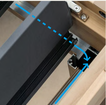
Sistema scarico acqua integrato Integrated water drainage system Système intégré d'écoulement de l'eau Integriertes Wasserablaufsystem Sistema integrado de descarga agua
